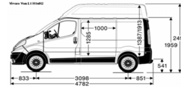
Vivaro Van L1 H1642
