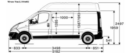
Vivaro Van L2 H1642
